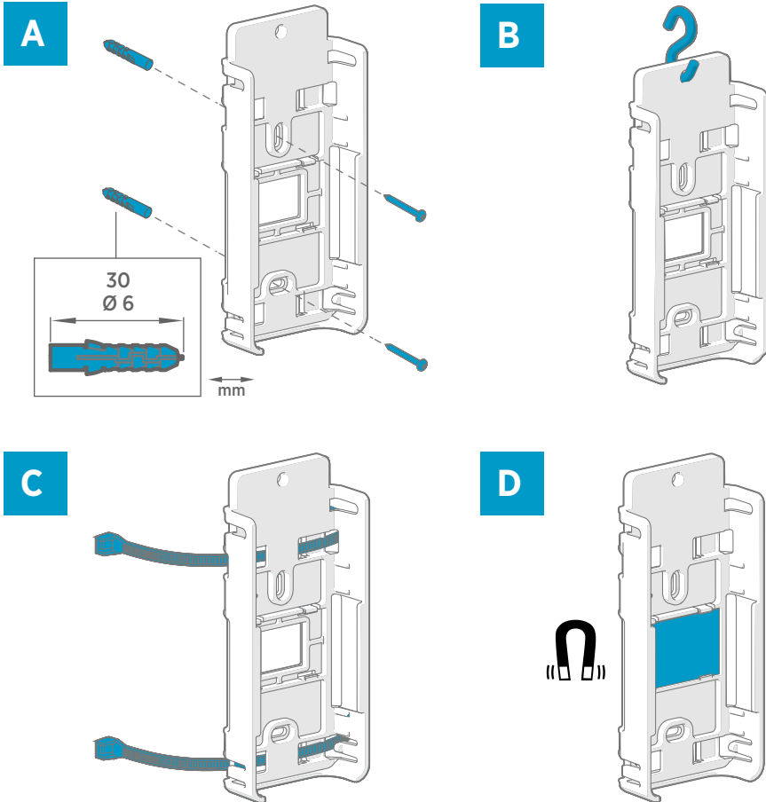
Kuva 2 CWL100:n kiinnitystavat
